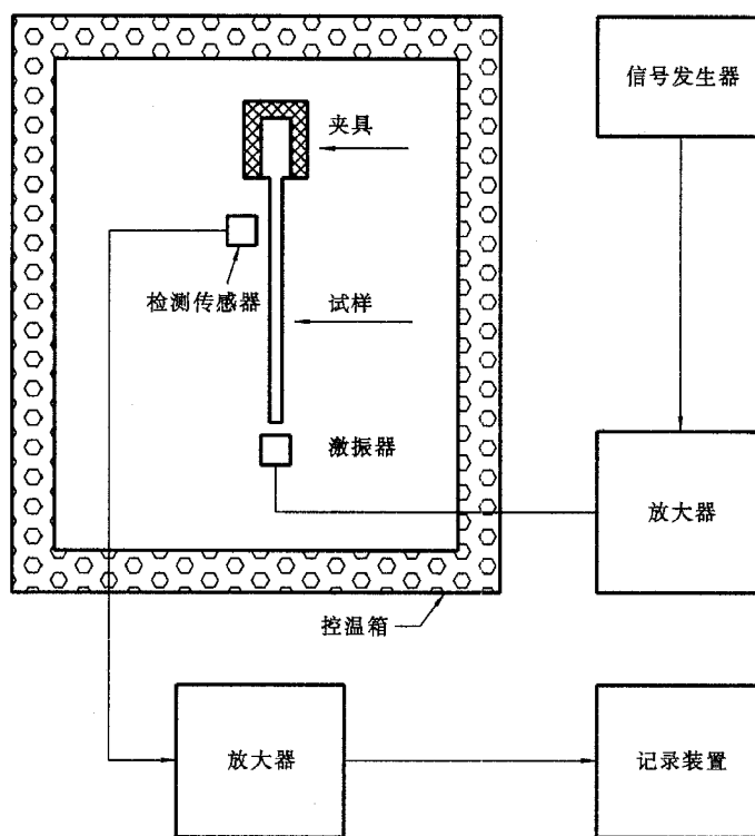
图 1 实验框图
